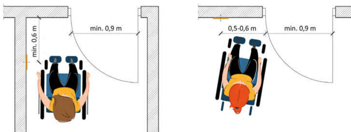
Ilustracja 33. Zasady lokalizowania domofonów oraz przycisków otwierających drzwi, rys. Katarzyna Guratowska i Maria Görlich-Opyd (opracowanie własne na podstawie „Modelu Dostępnej Szkoły”)
