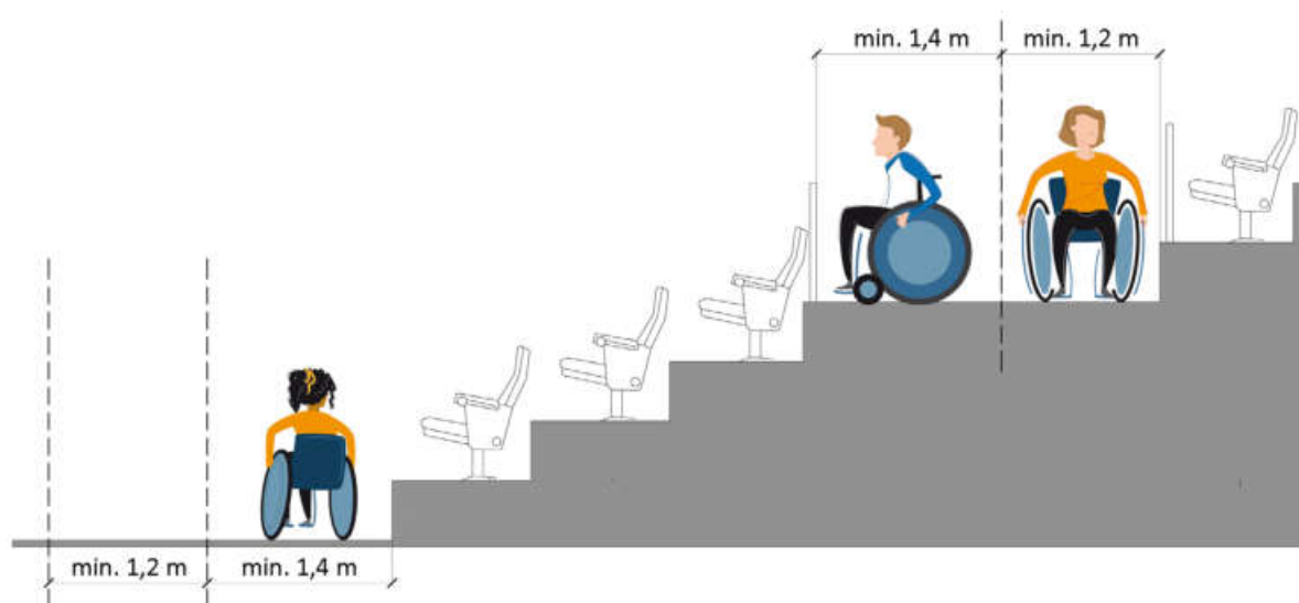
Ilustracja 94. Aranżacja miejsc dla osób na wózkach w obrębie widowni – przekrój, rys. Agnieszka Sowińska i Maria Görlich-Opyd
