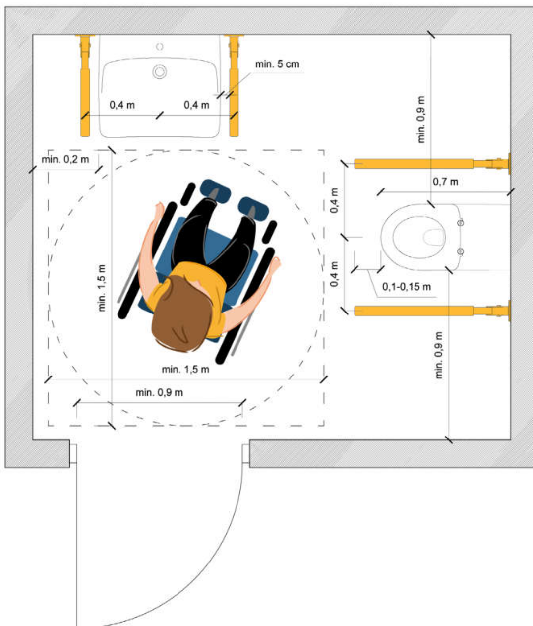
Ilustracja 77. Przykład rozmieszczenia sprzętów oraz powierzchni manewrowej i transferowej w toalecie przeznaczanej dla osób ze szczególnymi potrzebami, rys. Katarzyna Guratowska i Maria Görlich-Opyd (opracowanie własne na podstawie „Modelu Dostępnej Szkoły”)
