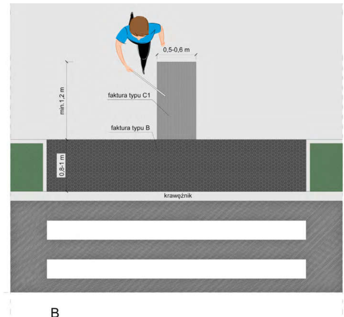
Ilustracja 26. Zasady stosowania pasów ostrzegawczych przy przejściach dla pieszych – przykład pasa ostrzegawczego zaczynającego się bezpośrednio za krawężnikiem, rys. Katarzyna Guratowska i Maria Görlich-Opyd
