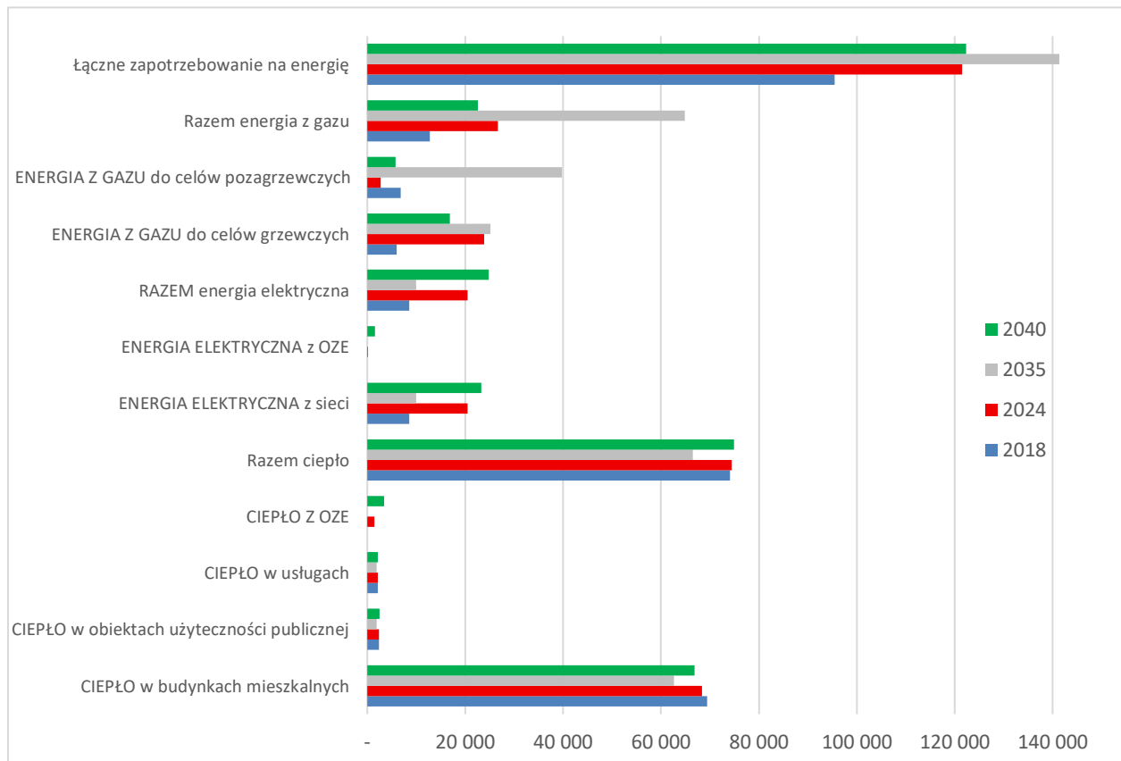
Rysunek 24 Przewidywane zmiany w zapotrzebowaniu na energię w Gminie Pszczółki od 2018 do 2040 roku
