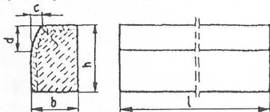
Rys. 1. Wymiarowanie krawężników
